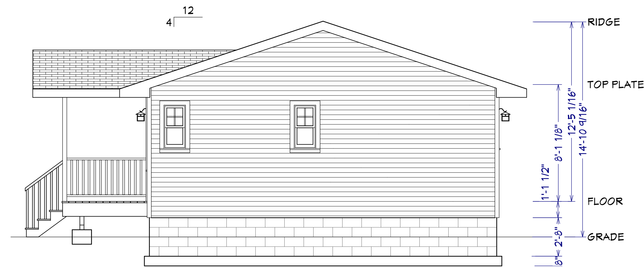
RIGHT ELEVATION SCALE: 1/4" = 1'
