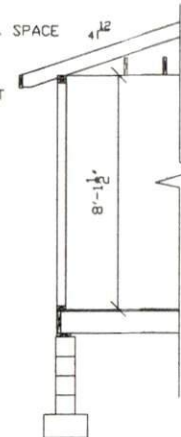
SCALE: 1/2"=1'
