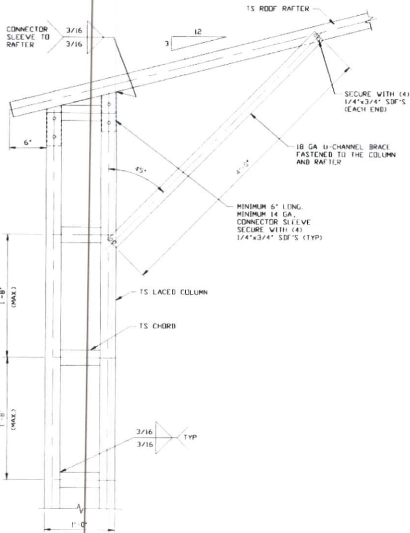
BRACE SECTION SCALE: NTS
