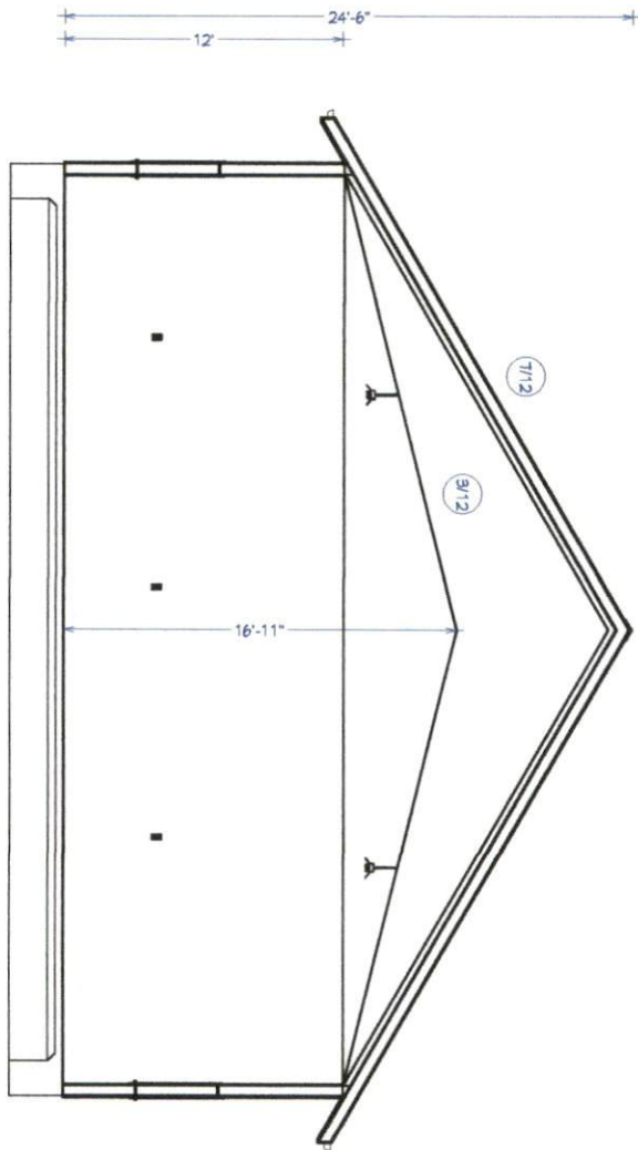
Elevation 1
