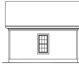
RIGHT ELEVATION SCALE: 1/4" = 1'-0"
