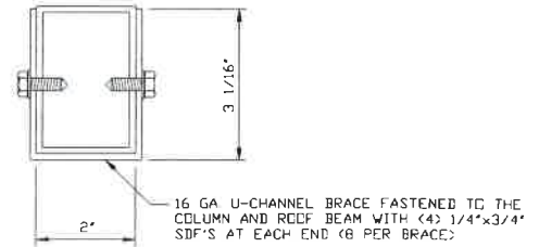
BRACE SECTION SCALE: NTS
