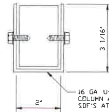
BRACE SECTION SCALE: NTS
