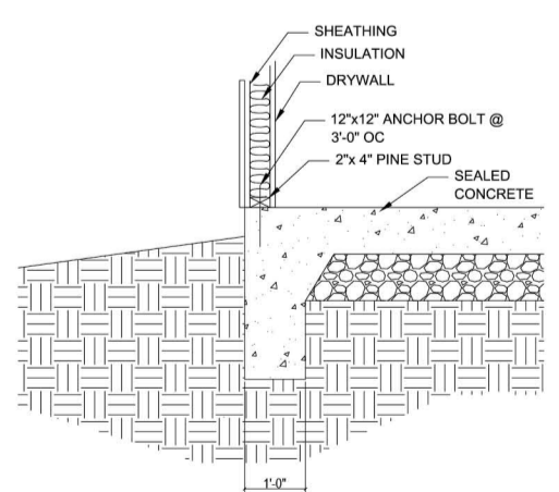
D1 SLAB DETAIL SCALE: \frac{3}{4} " = 1'-0"
