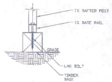
SECTION 1 SCALE: NTS (SK-16)
