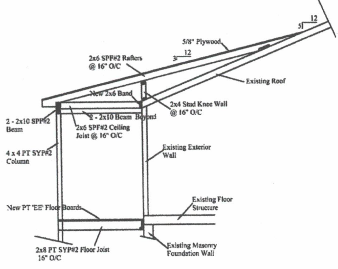
PORCH SECTION Scale: 1/4" = 1'-0"
