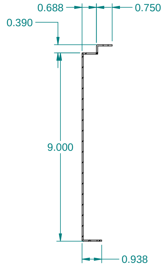
SECTION A-A
