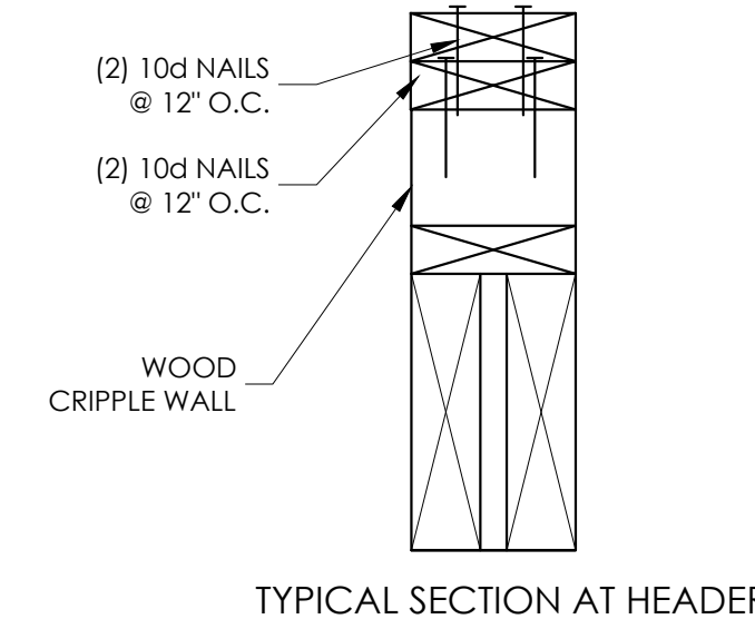
7 HEADER SECTION SCALE: NONE
