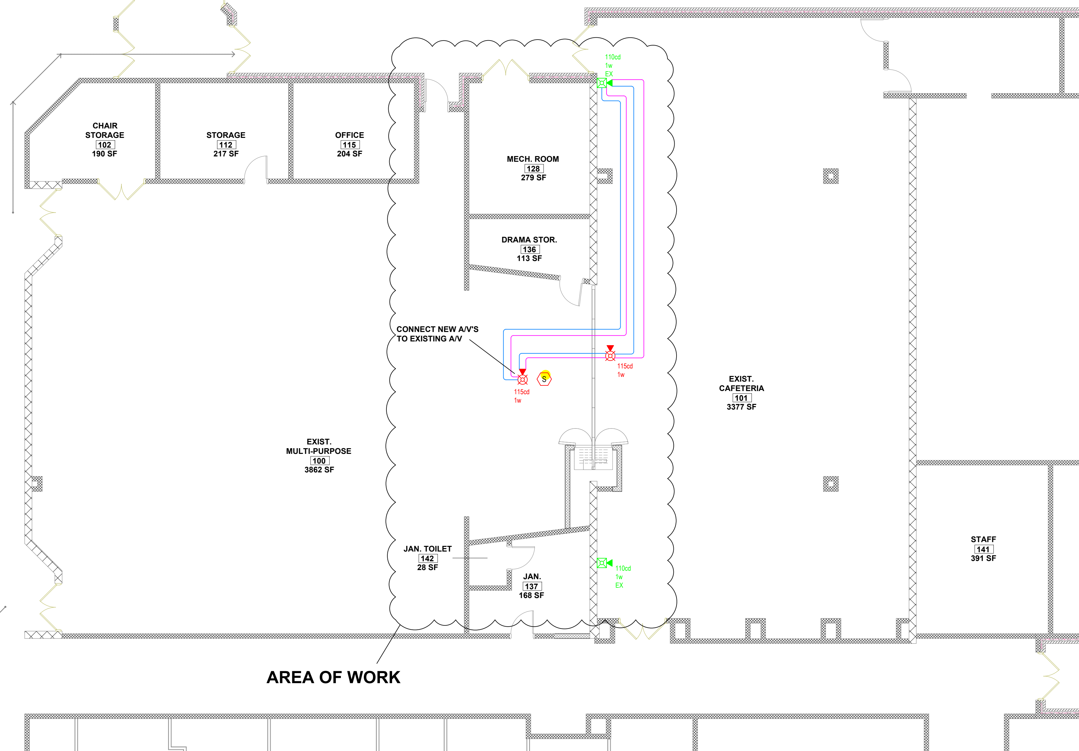
1 CAFETERIA EXPANSION FIRE ALARM SCALE: 1/8" = 1'0"
