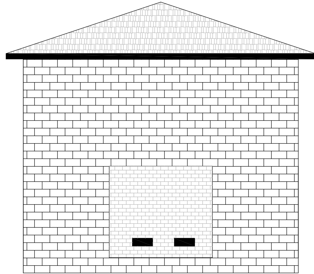
2 A-3 SIDE D ELEVATION SCALE: 3/16" = 1'-0"
