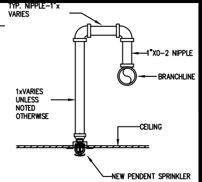
RETURN BEND DETAIL N.T.S.
