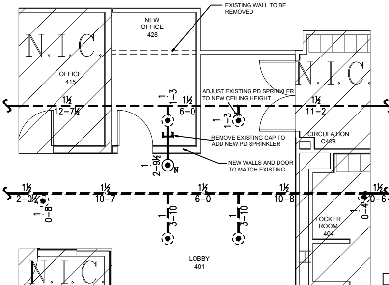
SPRINKLER PIPING PLAN SCALE: 1/8" = 1'-0"
