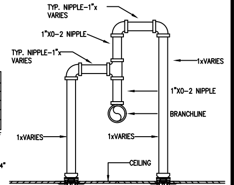
SPLIT RETURN BEND DETAIL N.T.S.
