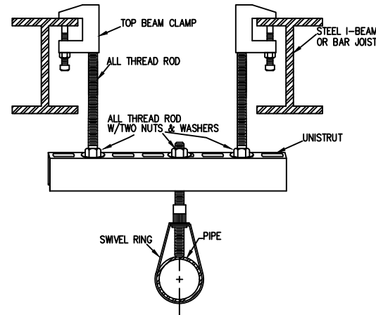
UNISTRUT HANGER DETAIL N.T.S.
